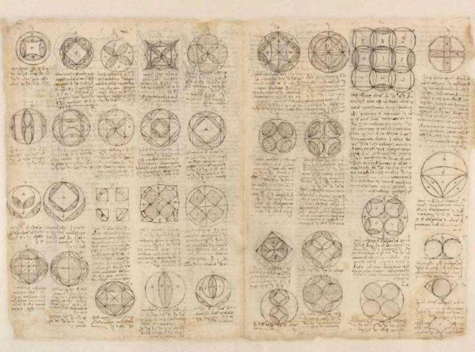
Codex Atlanticus : Répartition du cercle et de la quadrature (Fol. 471)
