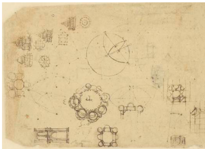
Codex Atlanticus : décomposition du cercle et quadrature (Fol. 1010)
